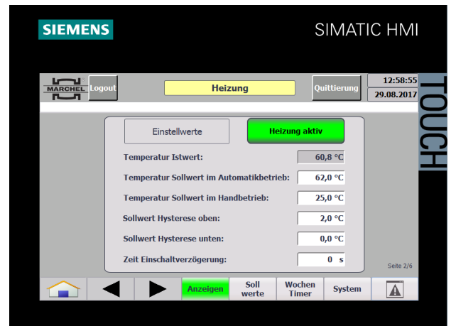
Ansicht Heizungsregelung
